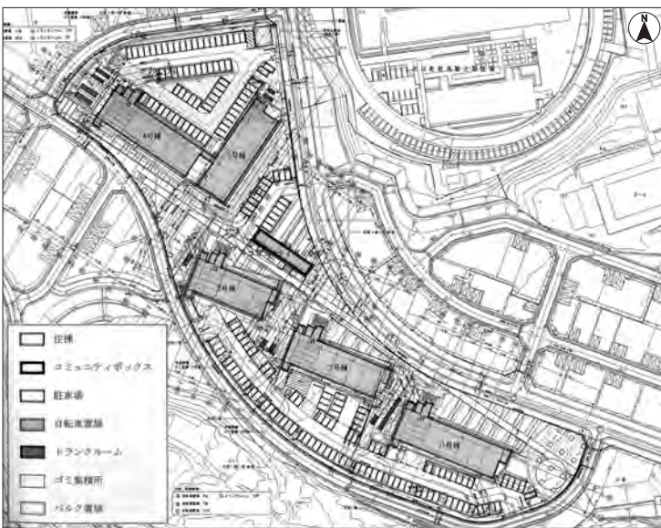
女川駅北地区災害公営住宅配置図
