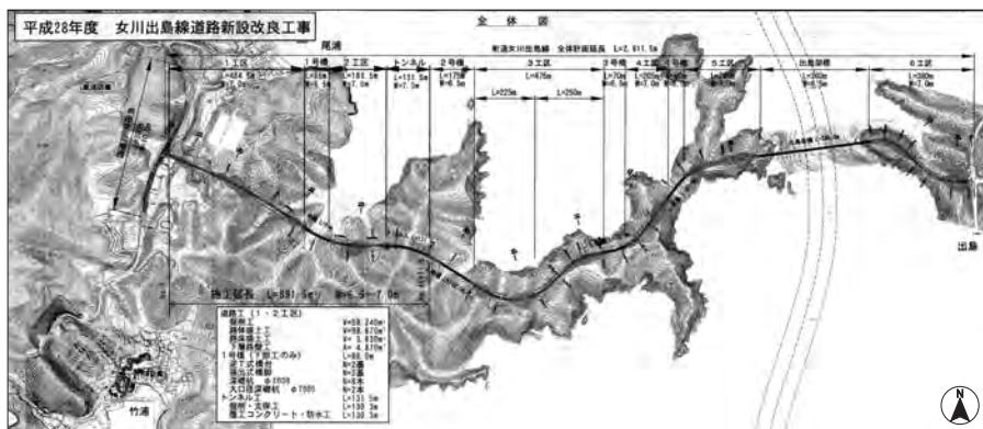
女川出島線道路新設改良工事予定図
